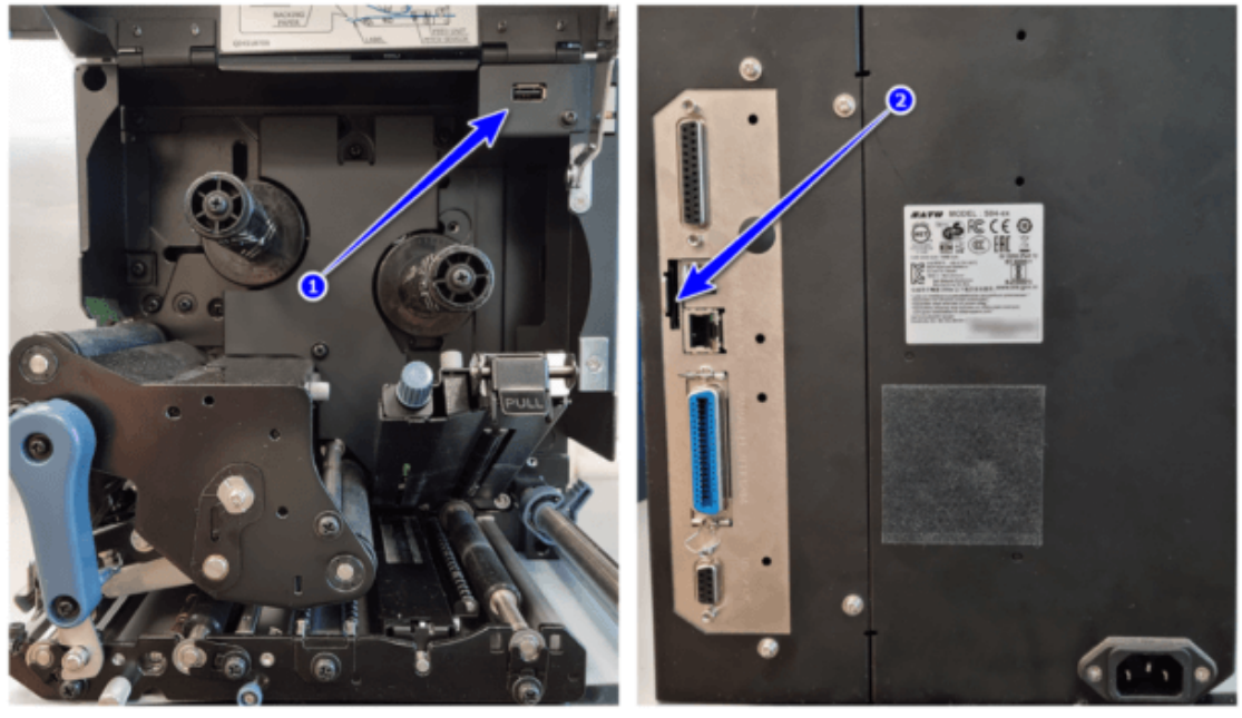
РАЗЪЕМЫ ДЛЯ ПОДКЛЮЧЕНИЯ ВНЕШНИХ НАКОПИТЕЛЕЙ НА ПРИВОДАХ SATO S84EX/S86EX 1 - РАЗЪЕМ РАЗЪЕМ ДЛЯ ПОДКЛЮЧЕНИЯ USB-ФЛЕШКИ 2 - РАЗЪЕМ ДЛЯ ПОДКЛЮЧЕНИЯ КАРТЫ ПАМЯТИ SD
